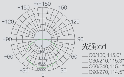
平均光束角 ( 50% ) : 115.0°
